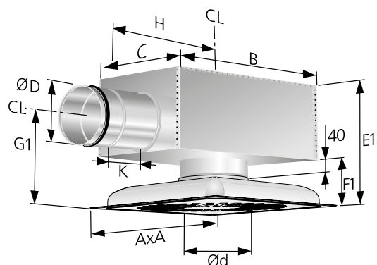
Kuva 5. SWIFT Ceiling.
