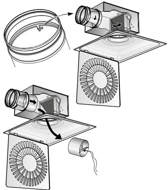
Kuva 3. Säättöpellin irrotus
