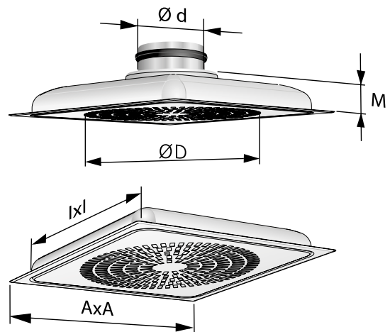
Kuva 5. LOCKZONE Ceiling.
