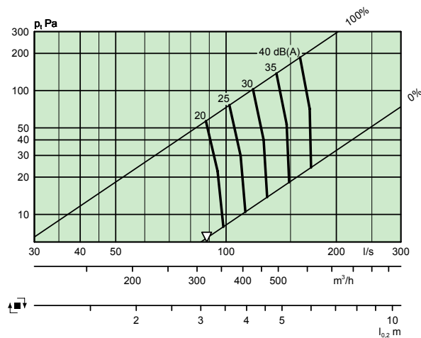
LOCKZONE C 315-600 + ALS 250-315 – Yksi mittamuutos
