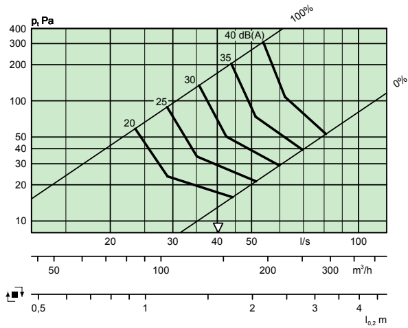
LOCKZONE C 200-500 + ALS 125-200 – Two steps
