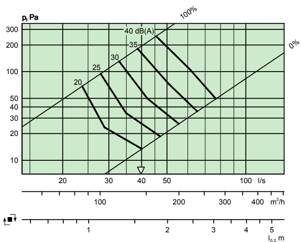
LOCKZONE C 200-600 + ALS 125-200 – Two steps
