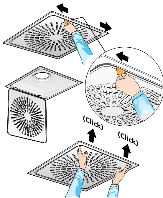
Figur 2. Quick Access, demontering av front.
