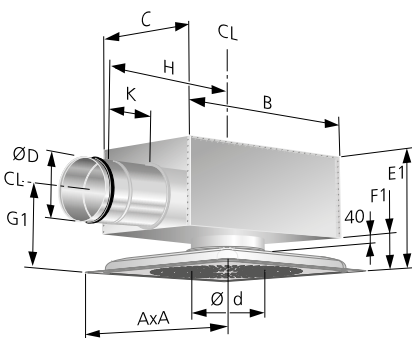
Figur 7. LOCKZONE C med ALS. CL = Centerline.
