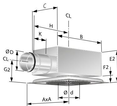
Figur 8. LOCKZONE C med ALS, låg bygghöjd.
