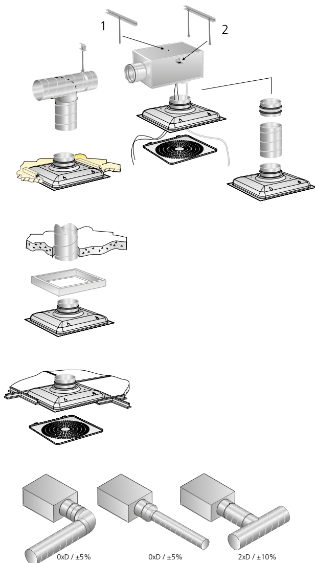
Figur 3. Monteringsalternativ.
