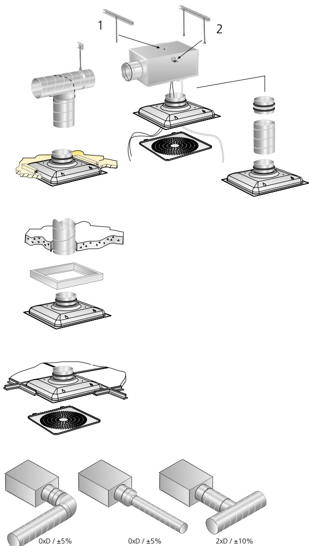
Abbildung 3. Montage.
