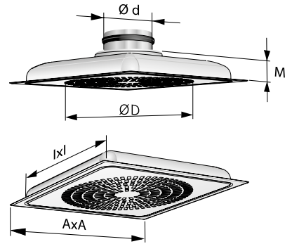
Abbildung 6. LOCKZONE Ceiling.
