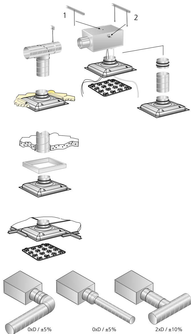
Figur 2. Monteringsalternativ.
