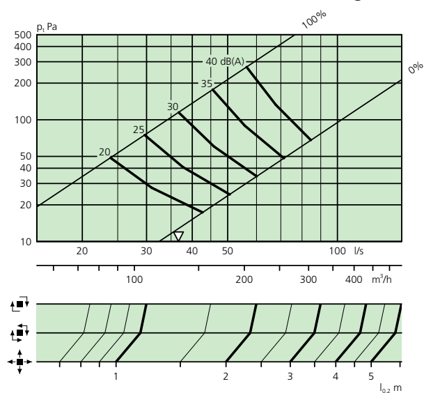
EAGLE CC 200-500 + ALS 125-200 - Två steg
