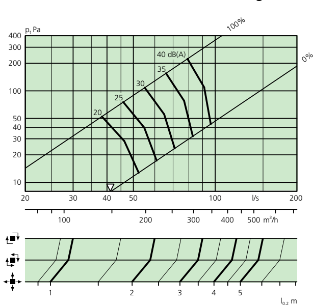
EAGLE CC 200-500 + ALS 160-200 - Ett steg
