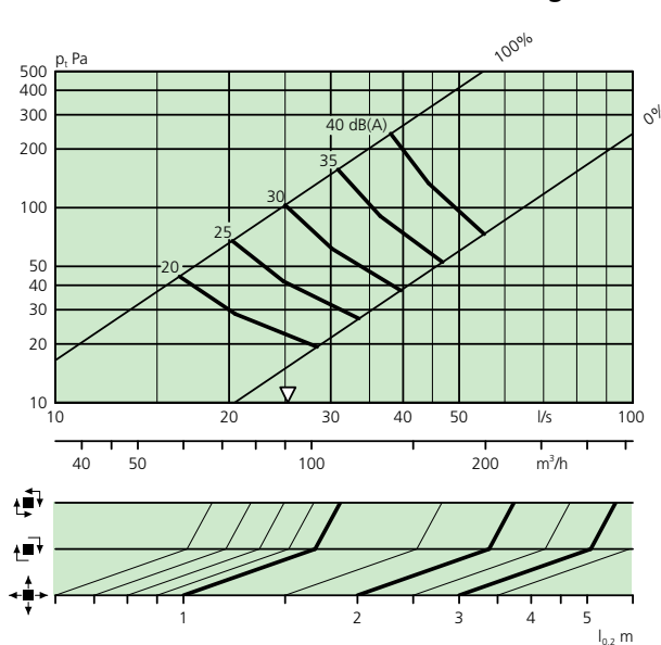
EAGLE CC 160-600 + ALS 100-160 - Två steg
