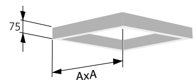
Abbildung 8. Rahmen, SAR K. Bei Größen 315-600 und 400-600 den Stützen des ALS-Kastens 20 mm über die Unterkante der Decke hinausragen lassen.
