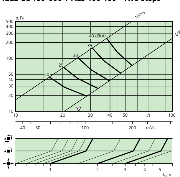
EAGLE CC 160-600 + ALS 100-160 - Two steps
