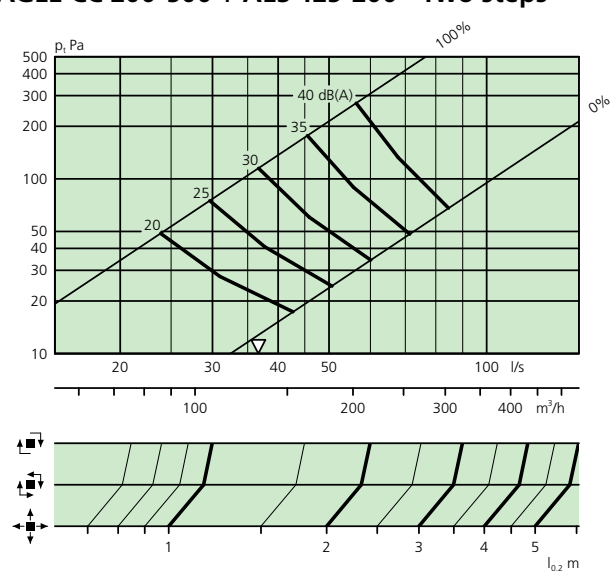
EAGLE CC 200-500 + ALS 125-200 - Two steps
