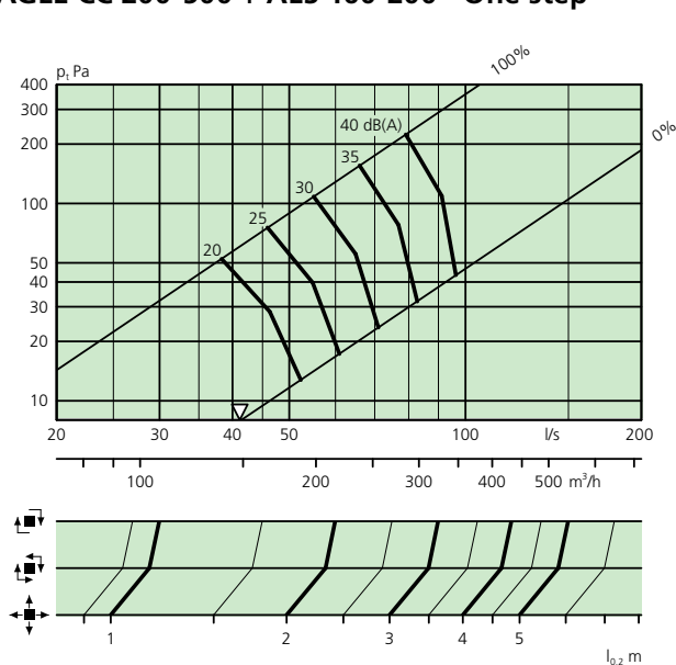
EAGLE CC 200-500 + ALS 160-200 - One step
