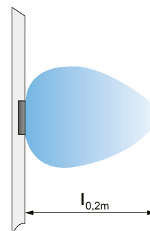
Figur 7. Isovel. Standard spredningsbillede, kort kastelængde (1V).
