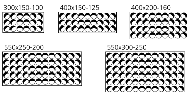
Figur 5. Standard dyseindstillinger, kort kastelængde (1V).
