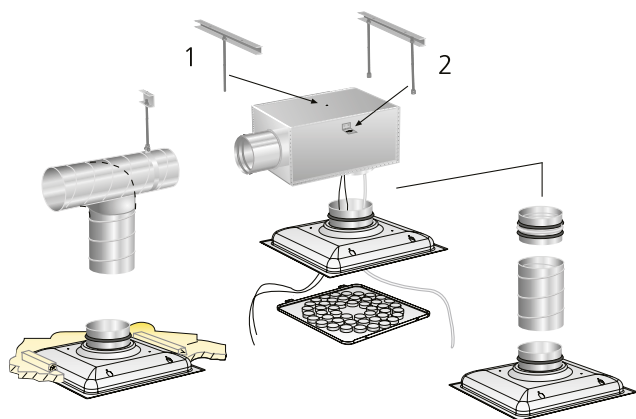
Figur 1. Quick Access, demontering av donfront.
