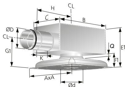
Figure 7. COLIBRI Ceiling avec ALS
