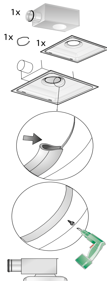
Figure 4. Installation des diffuseurs et du plénum d'équilibrage de hauteur réduite.
