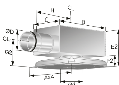
Figure 8. COLIBRI Ceiling avec ALS. Hauteur d'encastrement réduite.
