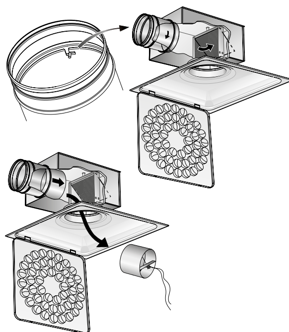
Figure 5. Le démontage du registre.
