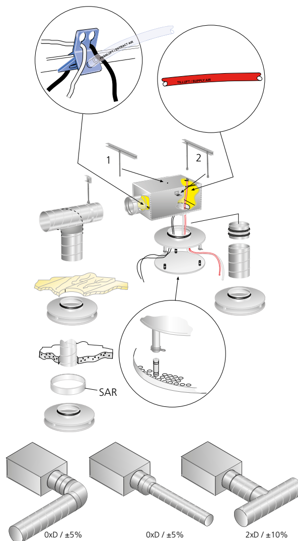
Figur 1. Montasje. Innregulering.
