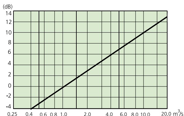
Diagram 2. Korrigering för andra luftflöden än 1 m 3 /s
