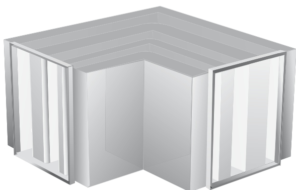
Figur 1. LARGO giver en jævn hastighedsfordeling efter bøjning- en ved at udnytte de akustiske lydbafler som ledeskinner.
