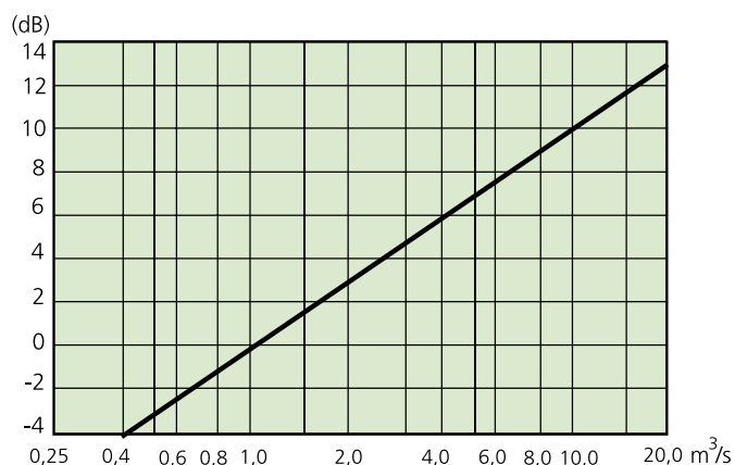
Diagram 2. Korrektion for andre luftmængder
