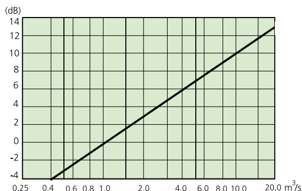
Diagram 2. Korrigerig för andra luftflöden
