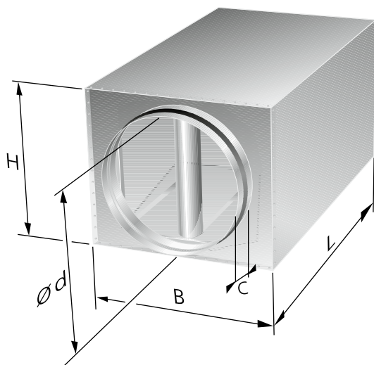
Figur 3 CLA-B – måttskiss
