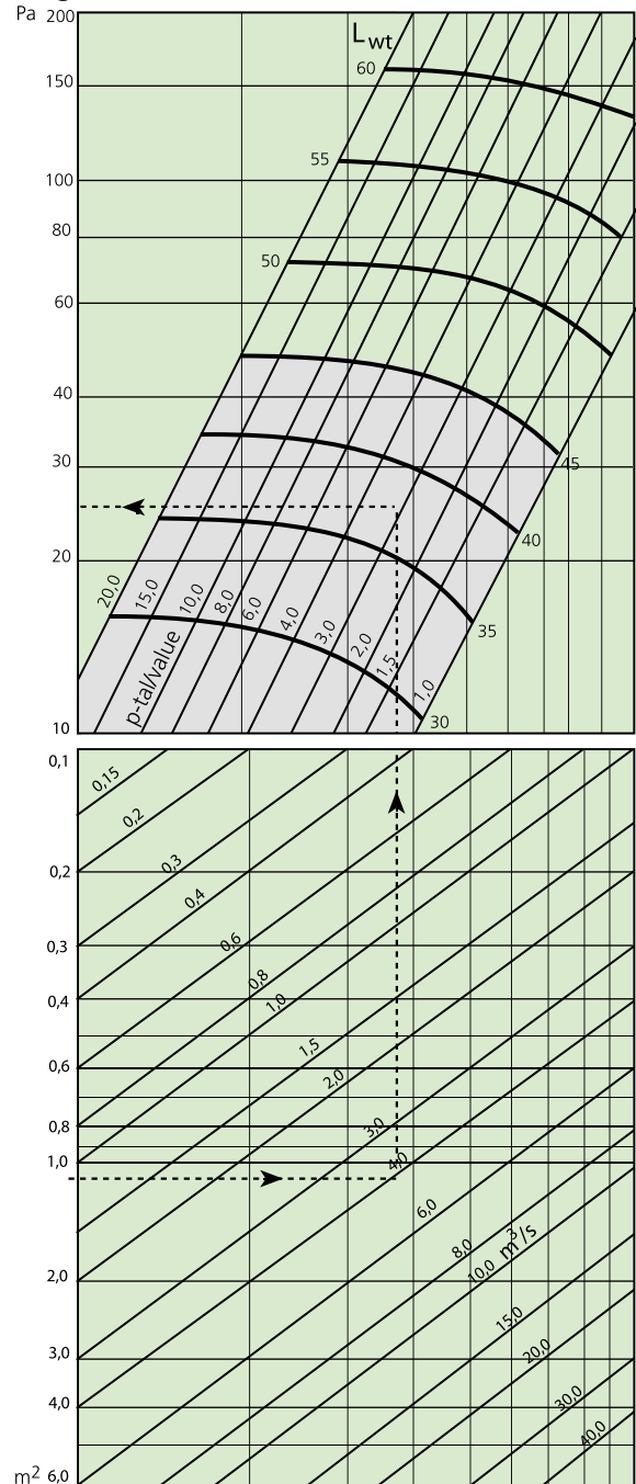
Nomogrammi 1. Painehäviön määrittäminen
