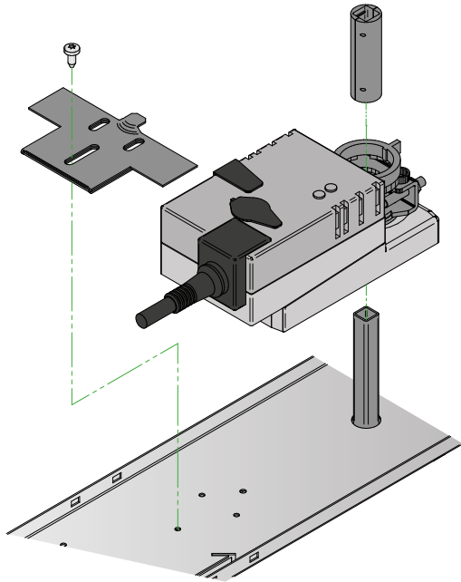
Abb. 13. Demontage des Klappenmotors.
