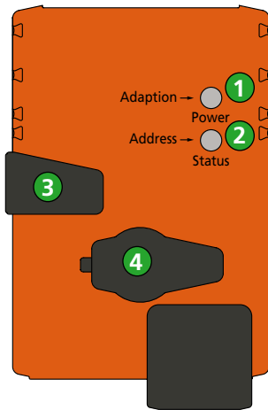
Abb. 10. Belimo-Stellantrieb.
