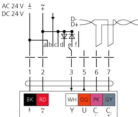
Abb. 9. Schaltplan.
