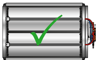
Abb 6. Montage - Für rechteckige Kanäle wird die Klappe immer so montiert, dass der Regler/Stellantrieb parallel zum Kanal montiert wird.
