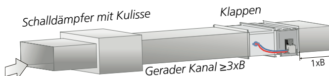
Abb. 8. Anforderungen an gerade Strecken 3 x B bei Schalldämpfern mit Kulissee. Gilt sowohl für Zu- als auch Abluft.
