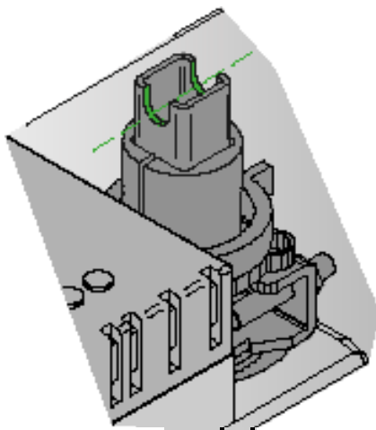
Abb. 14. Der Ausschnitt in der Klappenwelle zeigt die Stellung der Klappe an.
