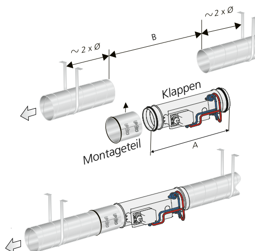
Abb. 4. Installation im Kanalsystem. Die Kanäle müssen in der Gebäudekonstruktion auf allen Seiten des Produkts fixiert werden.
