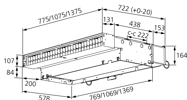
Figur 2. Måttskiss utan galler.
