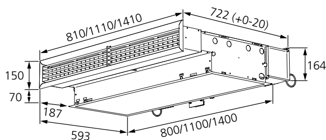
Figur 1. Måttskiss med galler.
