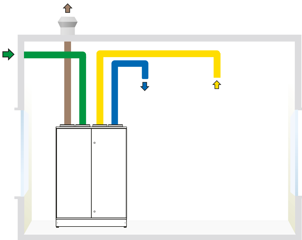
CASA W9 L, kanalanslutningar
