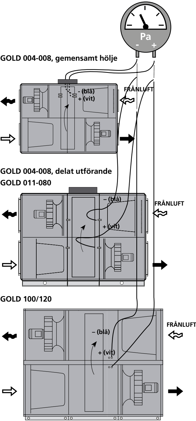
Tryckmätningar läckageriktning (Aggregat i högerutförande)
