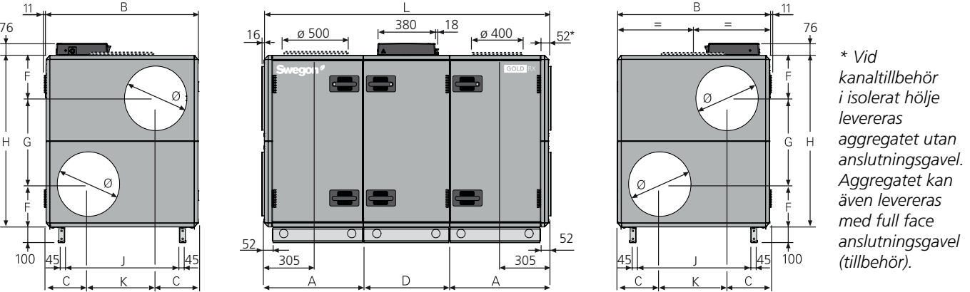
GOLD 007/008, delat utförande
