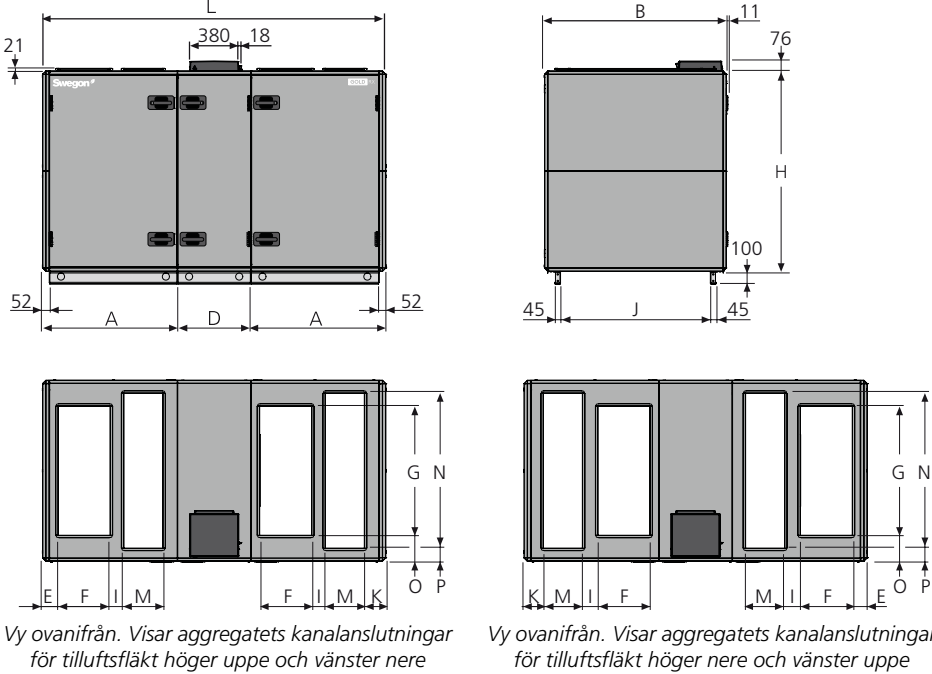
GOLD RX Top 014/020
