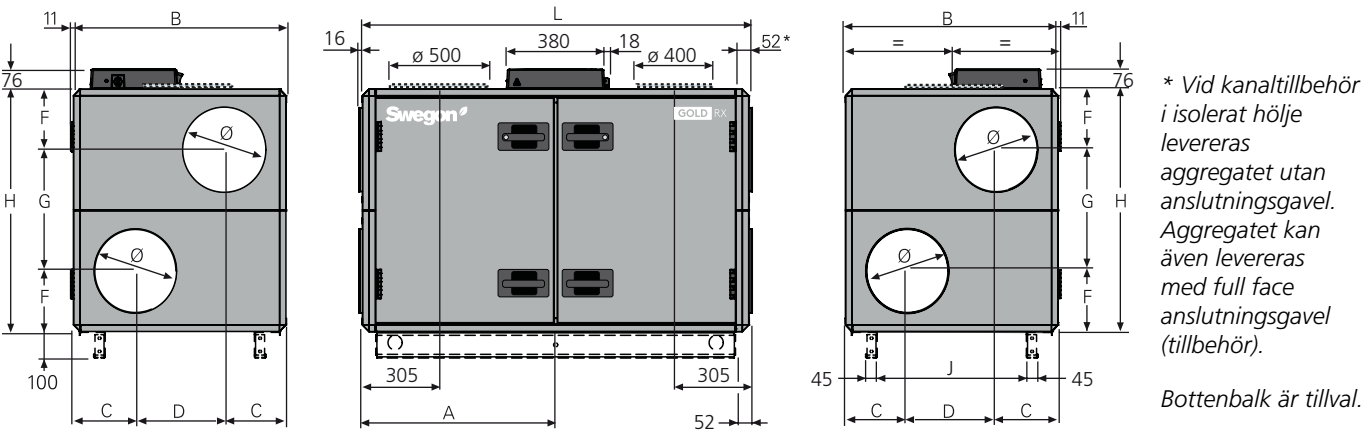
GOLD 007/008, gemensamt hölje
