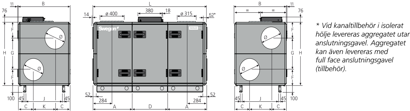
GOLD 007/008, delat utförande
