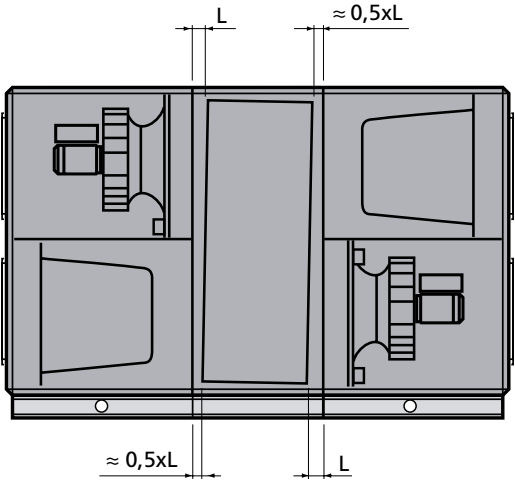
GOLD RX, storlek 050-120: skissen visar fabriksinställning av rotorns lutning vid fläktplacering 1. Lutningen skall alltid vara mot filter, vilket innebär att för fläktplacering 2 är lutningen åt andra hållet.
