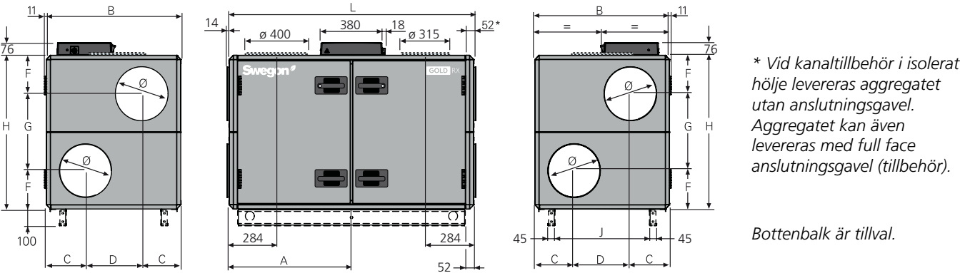
GOLD 004/005, gemensamt hölje
