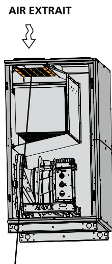
Plaques d'équilibrage Fixer les plaques d'équi- librage par emboîtement autour de la pièce de connexion du toit.
