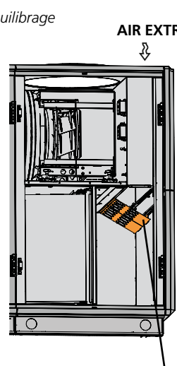
Plaque d'équilibrage Accrocher la plaque d'équilibrage dans l'encoche du côté du filtre. Soulever la plaque d'équilibrage vers le caisson de la CTA et l'accrocher dans l'encoche.
