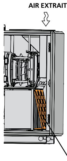
Plaque d'équilibrage Accrocher les plaques d'équilibrage sur le guide du filtre supérieur, puis enfoncer les plaques d'équilibrage vers le bas pour qu'elle se fixe dans le guide inférieur.
