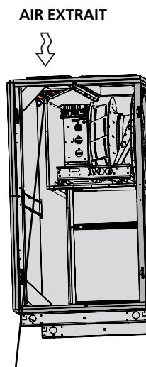
Plaques d'équilibrage Fixer les plaques d'équi- librage par emboîtement autour de la pièce de connexion du toit.
