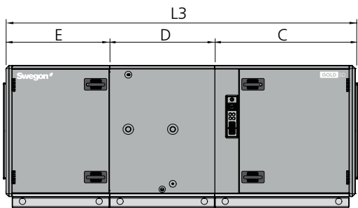
Vent. + Filtro + Intercamb. de calor de batería
