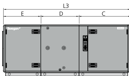
Ventilatore + filtro + rec. di calore a batteria
