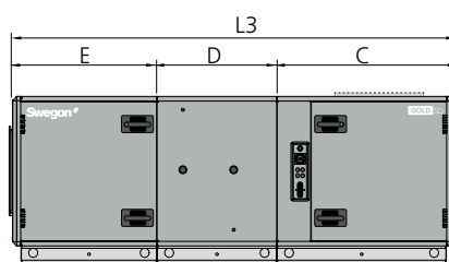
Ventilatore + filtro + rec. di calore a batteria
