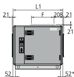
Ventilatore
