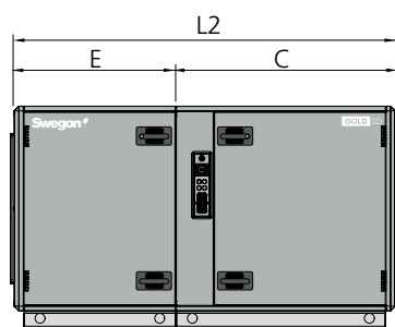
Ventilatore + filtro
