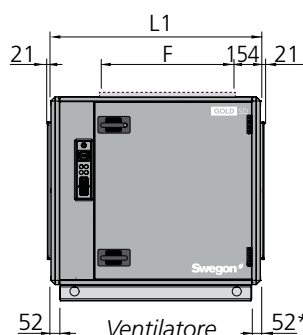
Ventilatore
