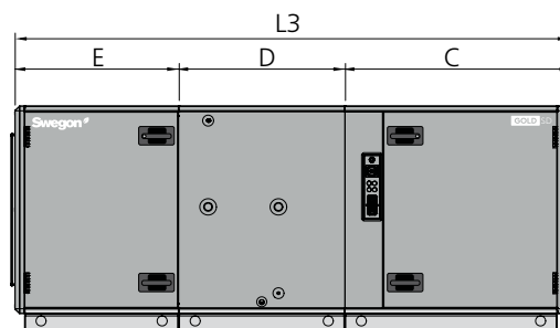
Puhallin + suodatin + patterilämmönsiirrin
