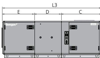
Puhallin + suodatin + patterilämmönsiirrin
