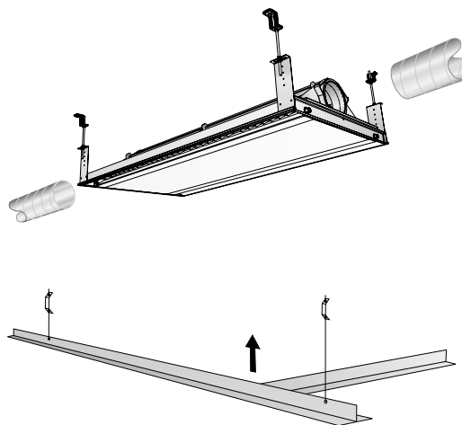
Figure 22. Installation de PACIFIC, ici suspendue au moyen de tiges filetées.
