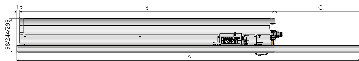
Figur 13. Måttskiss - fullstorlek
