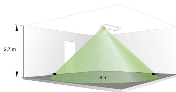
Figur 16. Detekteringsområde vid användning av sensormodul i underplåten
