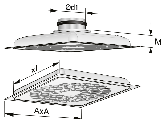
Rysunek 5. COLIBRI Ceiling.
