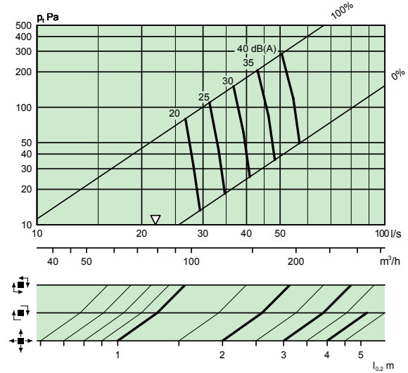
COLIBRI CC 160-600 + ALS 125-160 – 1 - stopień
