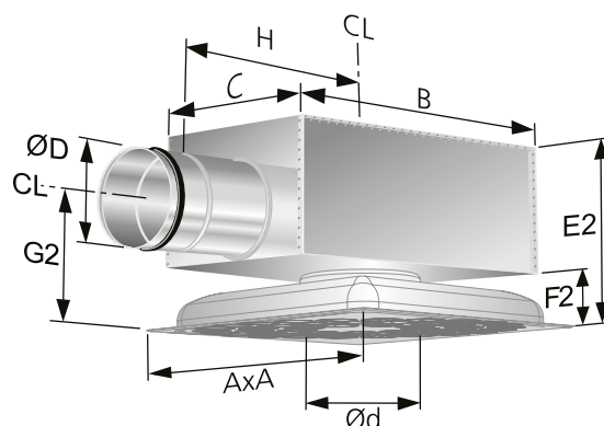
Rysunek 7. COLIBRI Ceiling z ALS. Wersja o obniżonej wysokości.
