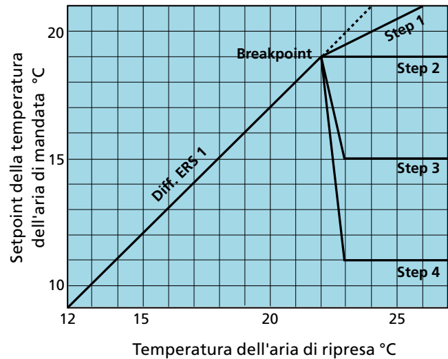
Regolazione ERS 1, esempio
