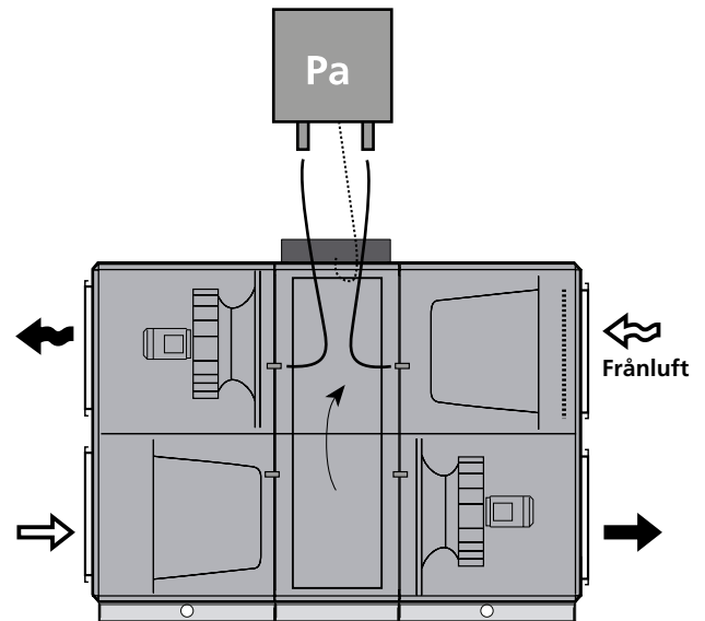
Princip för avfrostningsfunktion med separat tryckgivare.
