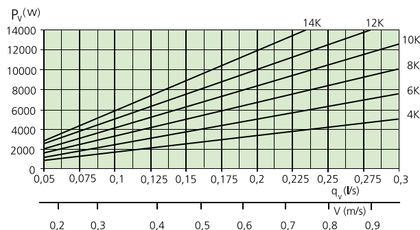
Diagram 5. Vattenflöde-värmeeffekt, per gren.
