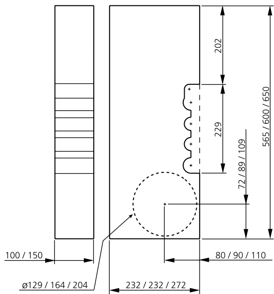
Figur 17. Väggblock WB.
