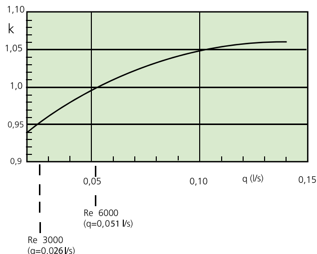
Diagram 3a. Vattenflöde-effektkorrektion
