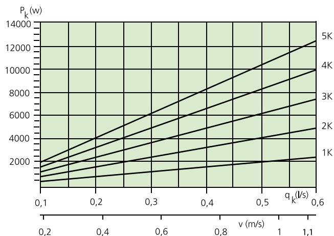
Diagram 2. Vattenflöde-kyleffekt, per gren.
