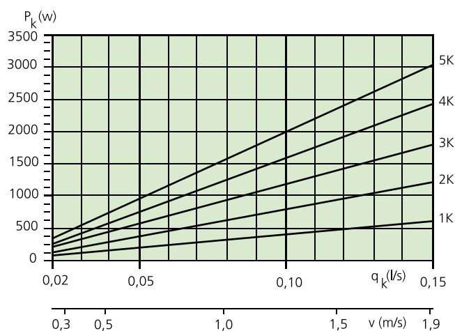
Diagram 1. Vattenflöde-kyleffekt, per apparat.
