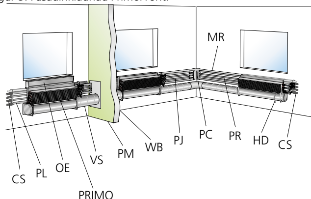
Figur 9. Fasadinklädnad PrimoFront.
