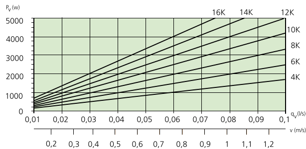
Diagram 4. Vattenflöde-värmeeffekt, per apparat.
