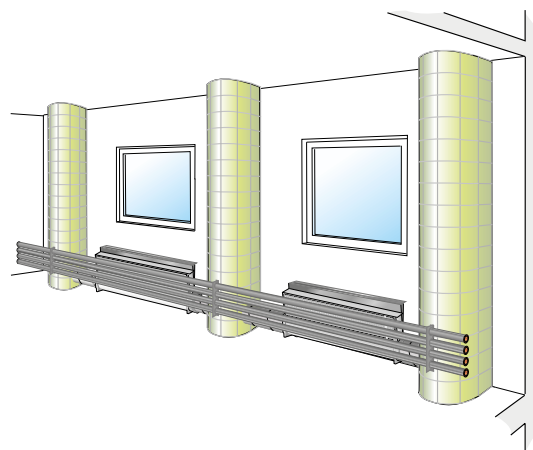
Figur 6. Primo med frontplacerade distributionsrör.
