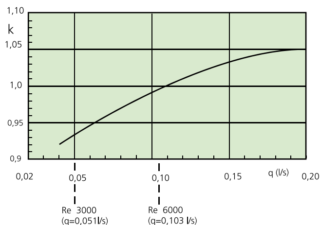
Diagram 3b. Vattenflöde-effektkorrektion
