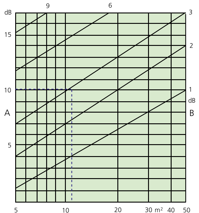
Diagram 6. Reduktionstal
