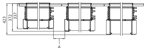
Figur 13. Monteringsutrymme. A = Min. monteringsavstånd 200 mm
