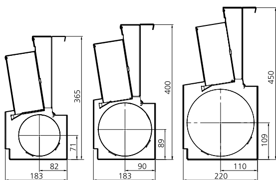
Figur 12. Vy: gavel. Ø125, Ø160 och Ø200
