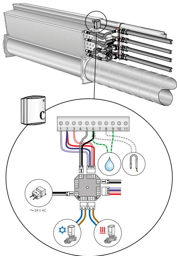
Figur 18. Styrutrustning LUNA. För inkoppling av elvärme, se separat monteringsanvisning på www.swegon.se
