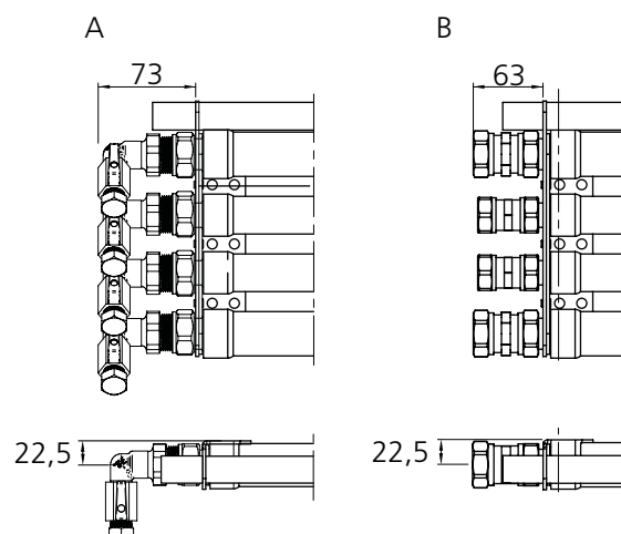
Figur 14. Anslutningsdetaljer. A = Röravslut, B = Rörinkoppling
