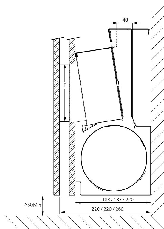
Figur 15. Sekundärluftöppning. Minimum avstånd mellan golv och inklädnad alternativt cirkulationsluftöppning i front panel. F = Format frontgaller 130 x apparatlängd (mm), där fri area är min. 49 %.
