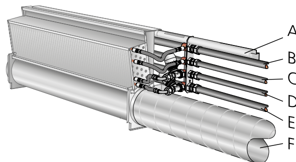
Figur 4. Anslutningsdimensioner..
