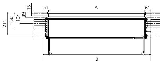
Figura 11. Vista frontale.
