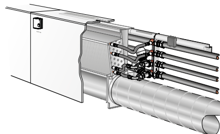
Figura 2. Installazione.
