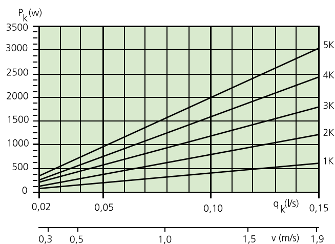
Diagramma 1. Portata d'acqua - potenza frigorifera per unità.
