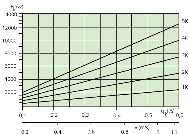
Diagramma 2. Portata d'acqua - potenza frigorifera per diramazione.
