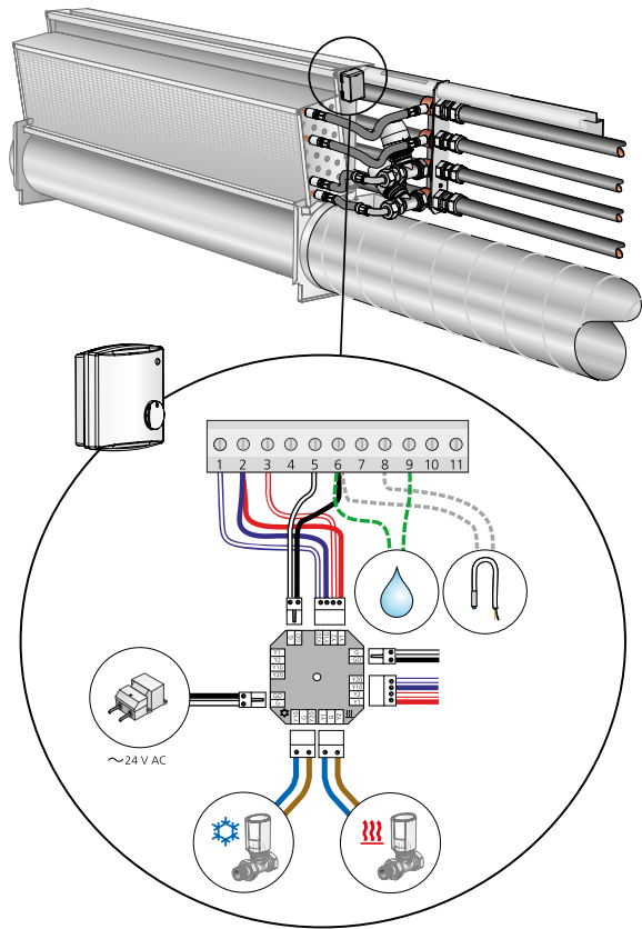
Figura 18. Dispositivo di controllo LUNA Per informazioni dettagliate sul collegamento del riscaldamento elettrico, fare riferimento alle istruzioni di installazione separate disponibili all'indirizzo www.swegon.com
