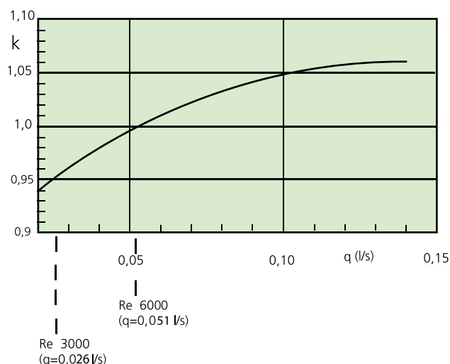
Diagramma 3a. Portata d'acqua - correzione della potenza
