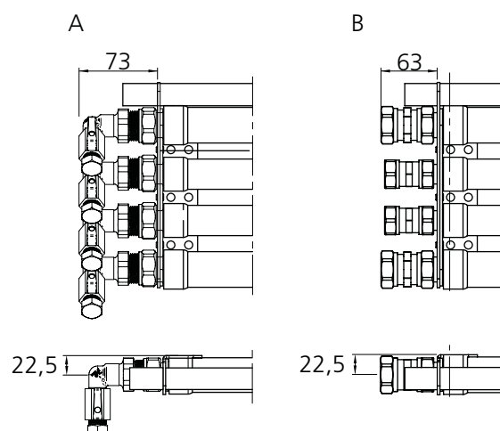
Figura 14. Componenti di collegamento.
