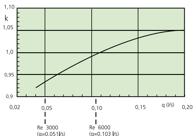
Diagramma 3b. Portata d'acqua - correzione della potenza
