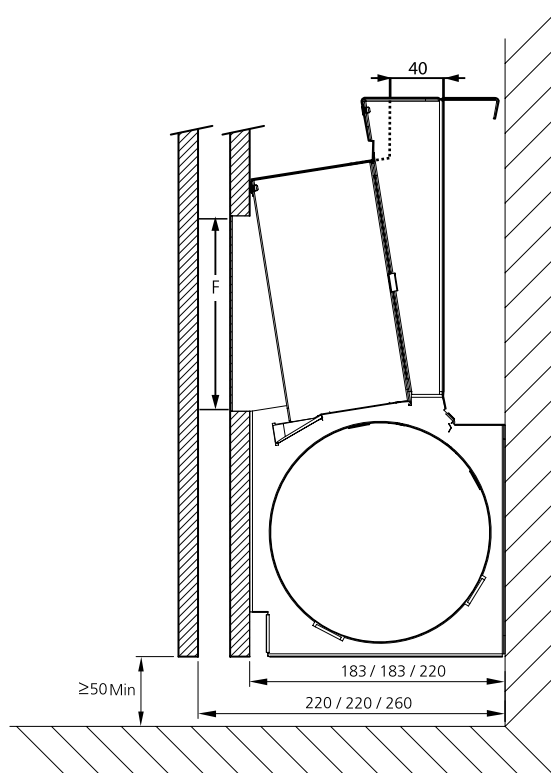
Figura 15. Apertura dell'aria secondaria. Distanza minima tra il pavimento e l'alloggiamento o l'apertura per il ricircolo dell'aria nel pannello frontale.
