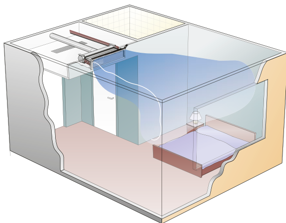
Figure 3. PRIMO monté au plafond dans les chambres d'hôtel.
