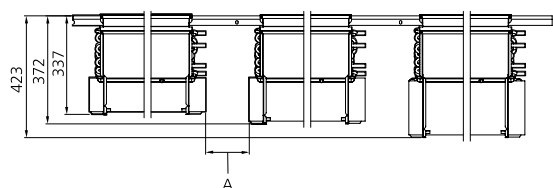
Figure 13. Encombrement. A=Distance mini. d'installation 200 mm
