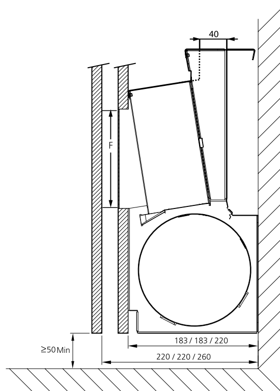
Figure 15. Ouverture air secondaire. Distance minimum entre le plancher et l'habillage ou l'ouverture pour l'air circulé dans le panneau frontal. F = Format de la grille frontale : 130 x longueur d'appareil, avec une surface libre d'au moins 49%.
