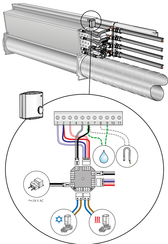
Figure 18. Appareil de commande LUNA. Pour les détails de câblage du chauffage électrique, voir les instructions d'installation sur www.swegon.com
