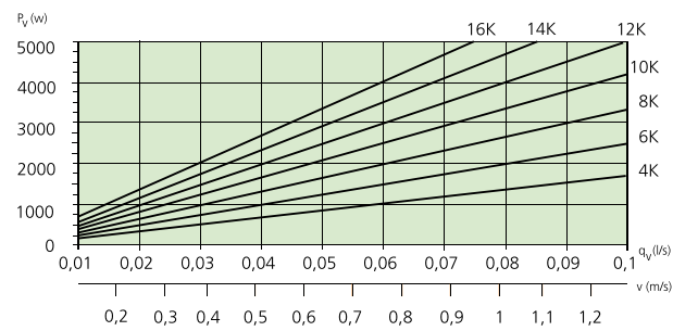
Diagramme 4. Débit d'eau – puissance de chauffage, par appareil
