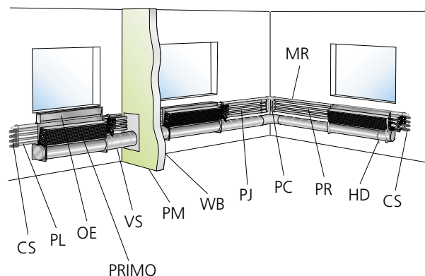
Figure 10. Repérage des accessoires.
