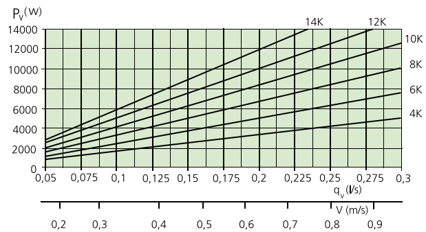
Diagramme 5. Débit d'eau – puissance de chauffage, par embranchement
