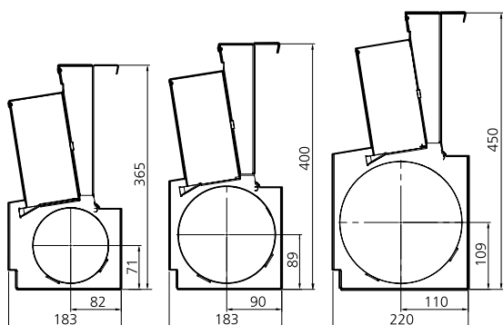
Figure 12. Vue : extrémité. Ø 125, Ø 160 et Ø 200
