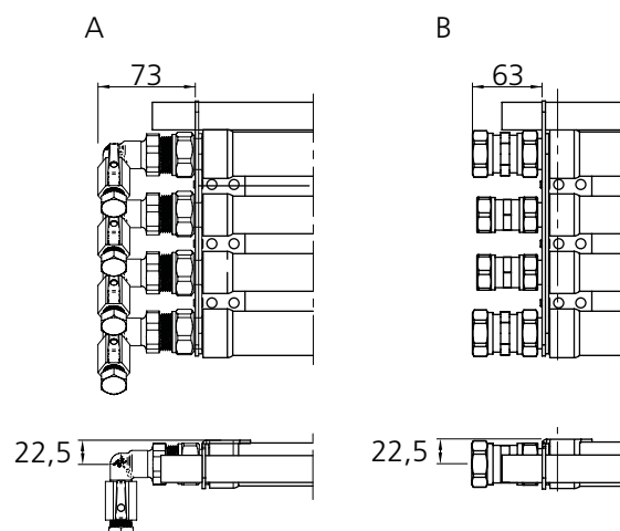
Figure 14. Pièces de raccordement. A=Terminaison de tuyau, B=Raccordement de tuyau
