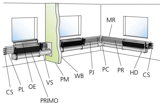
Kuva 10. Yhteenveto tarvikkeista.
