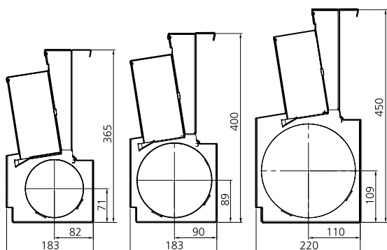
Kuva 12. Näkymä: päädystä. Ø 125, Ø 160 ja Ø 200
