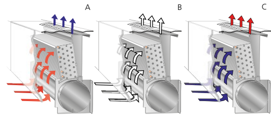
Kuva 1. Käyttötilat.
