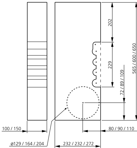
Kuva 17. Seinäkappale WB.
