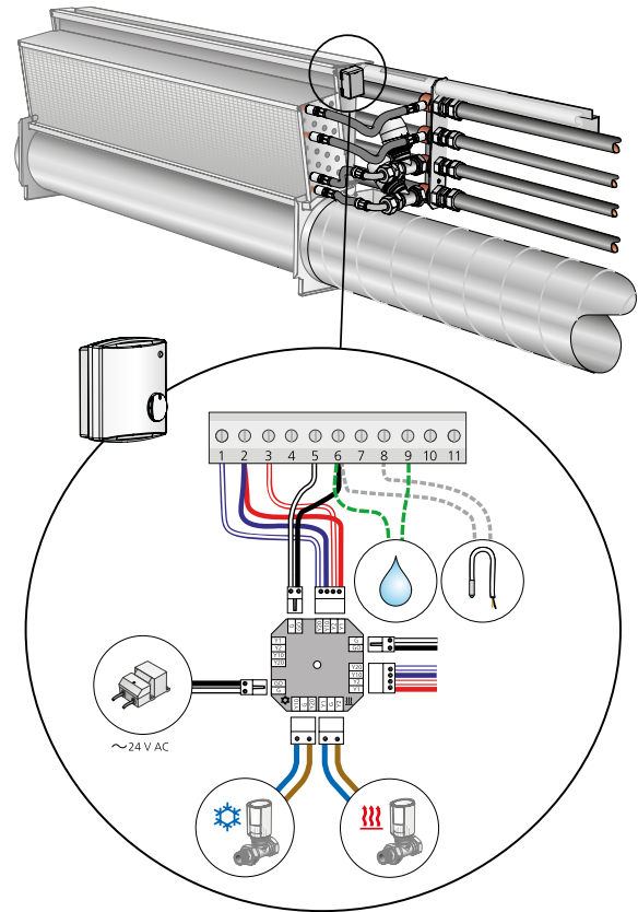
Kuva 18. Säätolaitte LUNA
