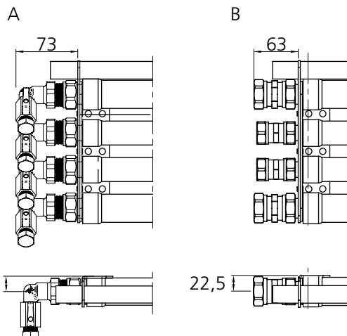
Kuva 14. Liitântätarvikkeita.
