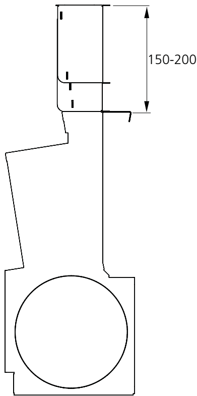
Kuva 16. Liitäntäkehys.
