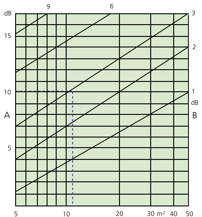
Käyrästä 6. Reduktiokerroin
