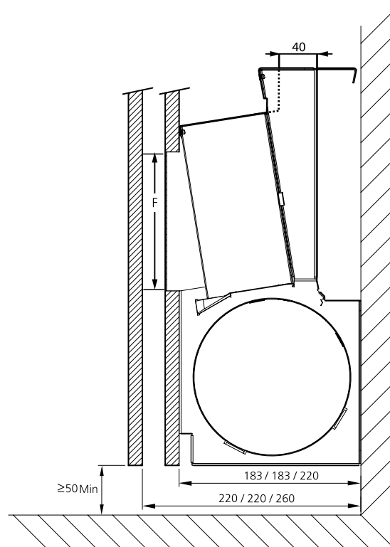
Kuva 15. Toisio-ilma-aukko.
