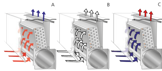
Abbildung 1. Betriebspositionen.
