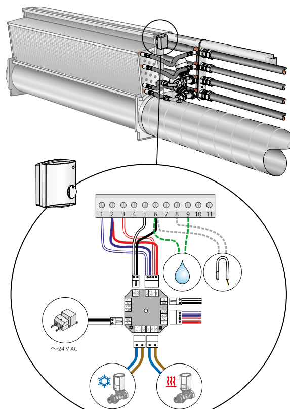
Abbildung 18. Steuerungsausrüstung LUNA. Für den Anschluss der Elektroheizung, siehe separate Montageanweisung auf www.swegon.com
