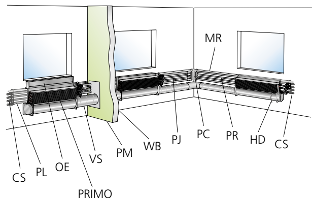
Abbildung 10. Zusammenstellung, Zubehör.
