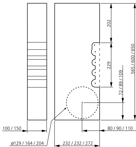
Abbildung 17. Wandblock WB.
