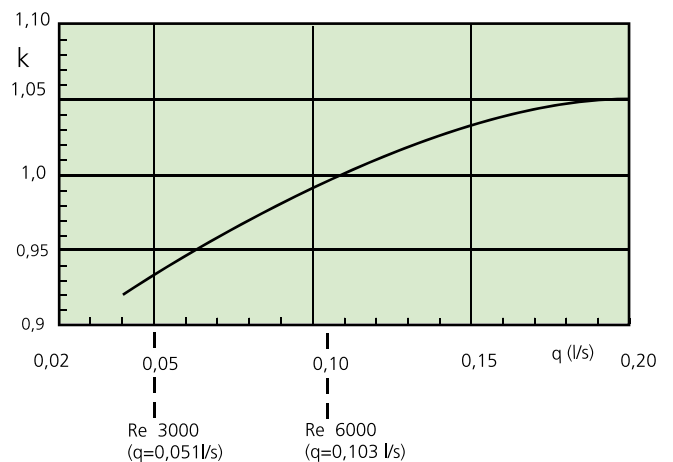
Diagramm 3b. Wassermenge – Leistungskorrektur
