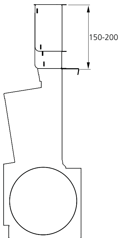
Abbildung 16. Auslassstutzen.
