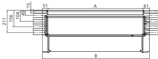
Abbildung 11. Vorderansicht. A = Auslassstutzen, B = Länge
