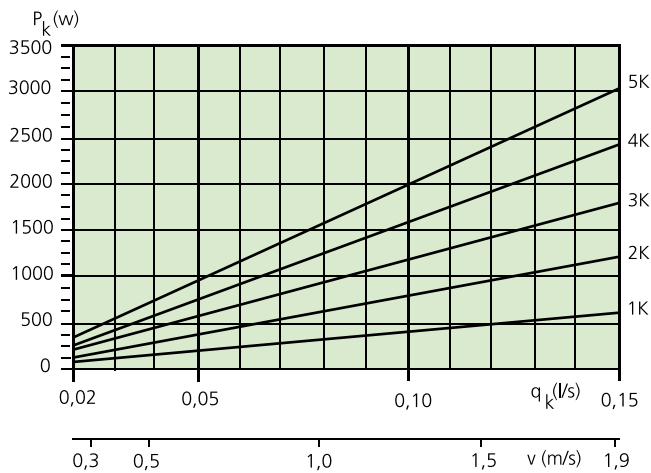
Diagramm 2. Wassermenge – Kühlleistung, pro Abzweig.
