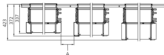
Abbildung 13. Platz für Montage. A = kleinster Montageabstand 200 mm
