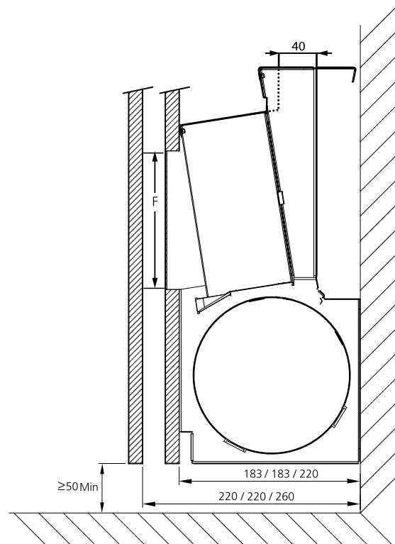
Abbildung 15. Sekundärluftöffnung. Der Minimumabstand zwischen Boden und Verkleidung oder Zirkulationsöffnung im Frontpaneel. F = geformtes Frontgitter 130 x Gerätelänge (mm), wo die freie Fläche mindestens 49 % beträgt.
