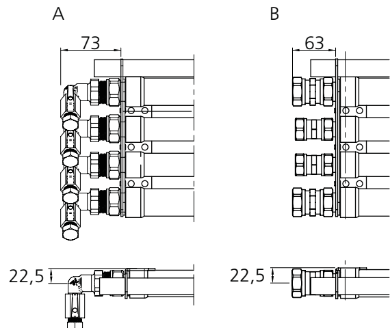
Abbildung 14. Anschlusssteile. A = Rohrabschluss, B = Rohranschluss
