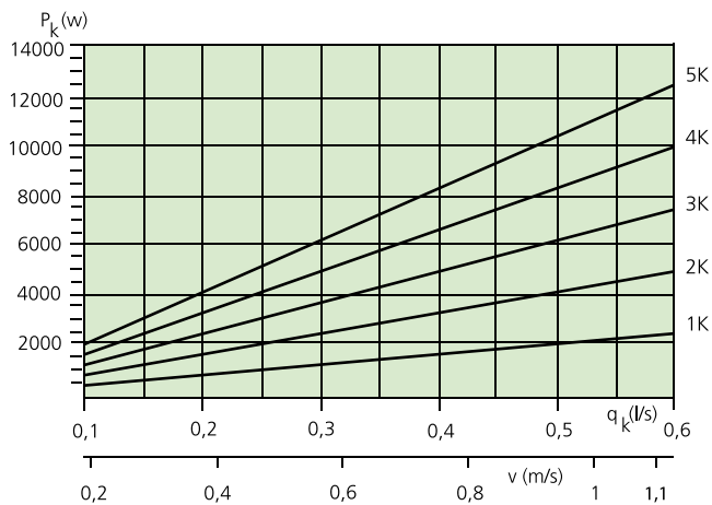
Diagramm 2. Wassermenge – Kühlleistung, pro Abzweig.
