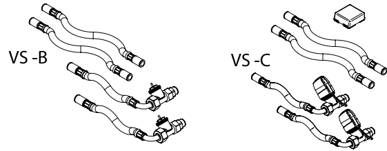
Abbildung 7. Ventilsatz VS
