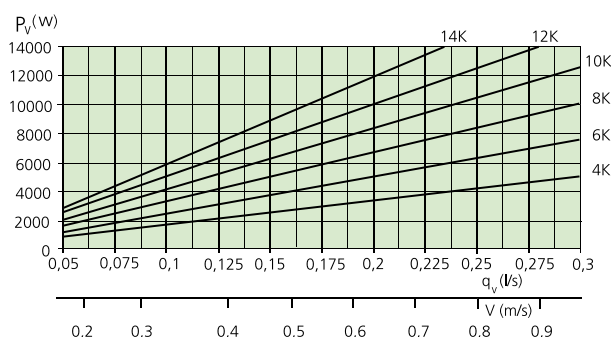
Diagramm 5. Wassermenge – Heizleistung, pro Abzweig.
