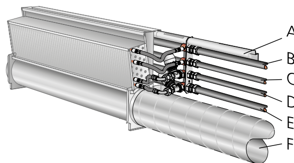
Abbildung 4. Anschlussabmessungen.. A. Steuerkabel, Verlegungsrohr Ø25 mm B. Rücklauf Kühlung, Ø28 mm C. Rücklauf Heizung, Ø22 mm D. Vorlauf Heizung, Ø22 mm E. Vorlauf Kühlung, Ø28 mm F. Luftkanal Ø125, 160 oder 200 mm
