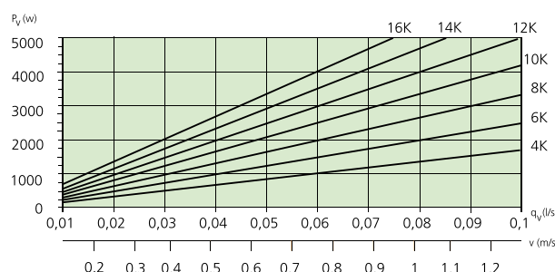
Diagramm 4. Wassermenge – Heizleistung, pro Gerät.
