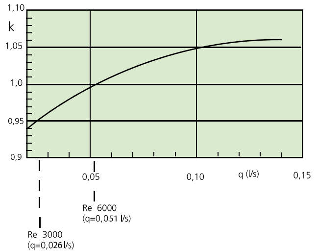
Diagramm 3a. Wassermenge - Leistungskorrektur
