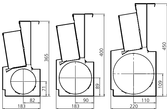
Abbildung 12. Ansicht: Endstück. Ø 125, Ø 160 ja Ø 200
