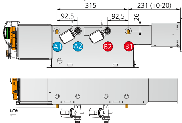
Kuva 23. Mitat vesiliitântä
