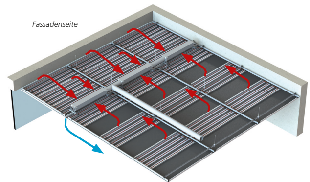
Strömungscharakteristik der Zuluft: Der Zuluftstrahl erzeugt einen Unterdruck im Deckenhohlraum, welcher warme Luft aus dem Raum durch die fassadenseitigen und den zwischen den Deckenplatten liegenden Fugen anzieht und per Umluft-Effekt abgekühlt in den Raum zurückführt.
