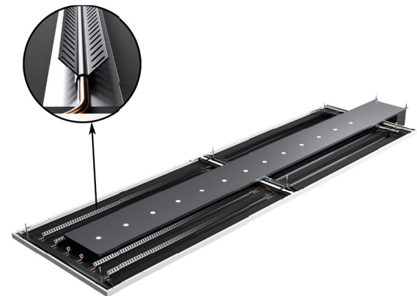
Opzionalmente più prestazioni: Convector Wings
