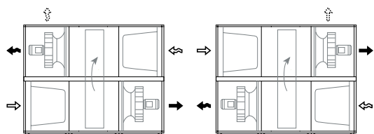
Tilluftsfläkt, höger, nere Tilluftsfläkt, höger, uppe Högerutförande
