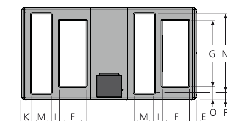
Vy ovanifrån. Visar aggregatets kanalslutningar för tilluftsfläkt höger nere och vänster uppe
