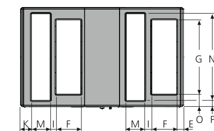
Vy ovanifrån. Visar aggregatets kanalslutningar för tilluftsfläkt höger nere och vänster uppe
