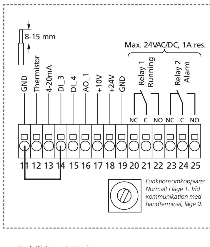
Fig. 1. Plintar i motorstyrning
