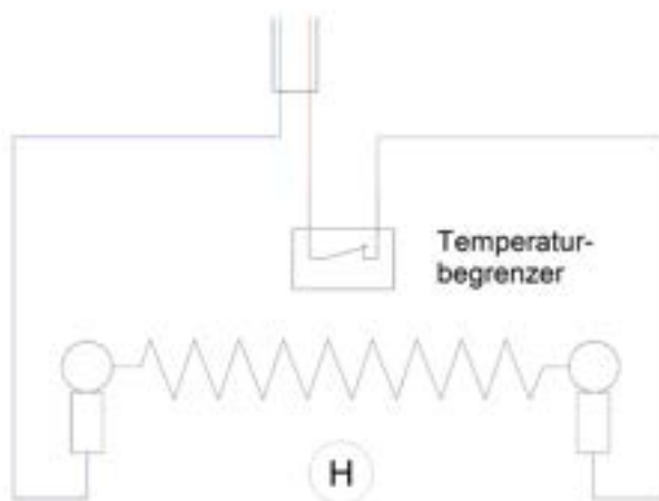
Elektroschema Heizung
