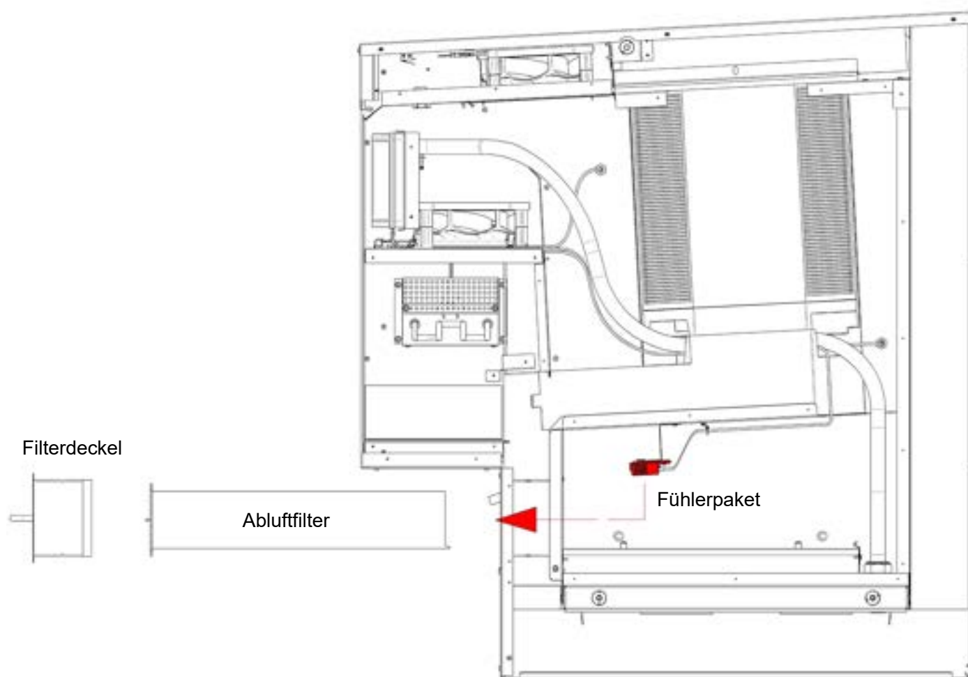
Abbildung 13: Austausch Fühlerpaket
