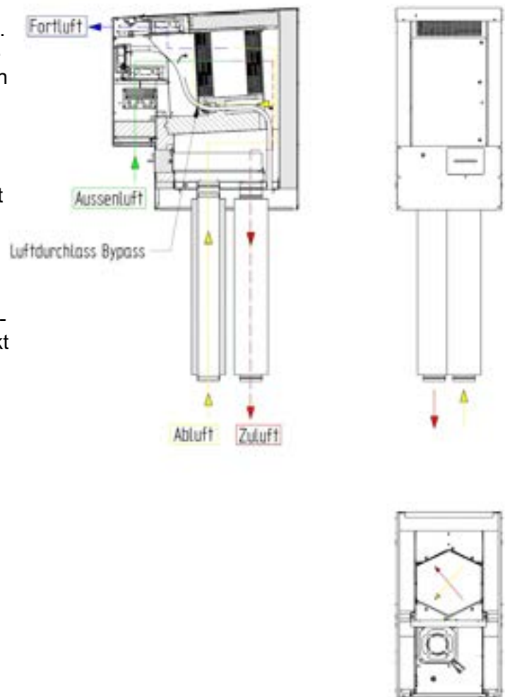
Abbildung 2: Luftwege
