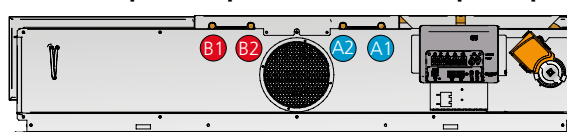
Figura 21. Raccordo per l'acqua sul bordo posteriore (WB).
