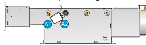
Figura 20. Raccordo per l'acqua sul lato sinistro.
