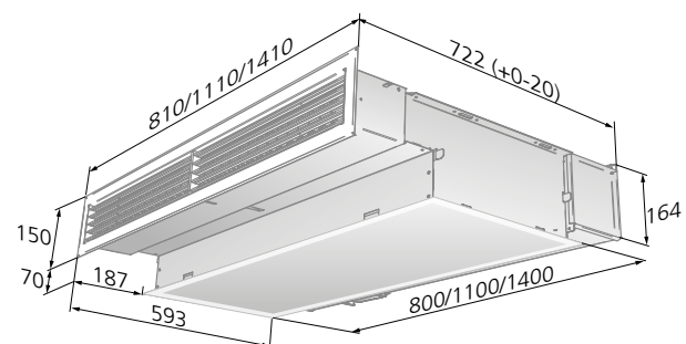
Figura 23. Schema delle quote con griglia
