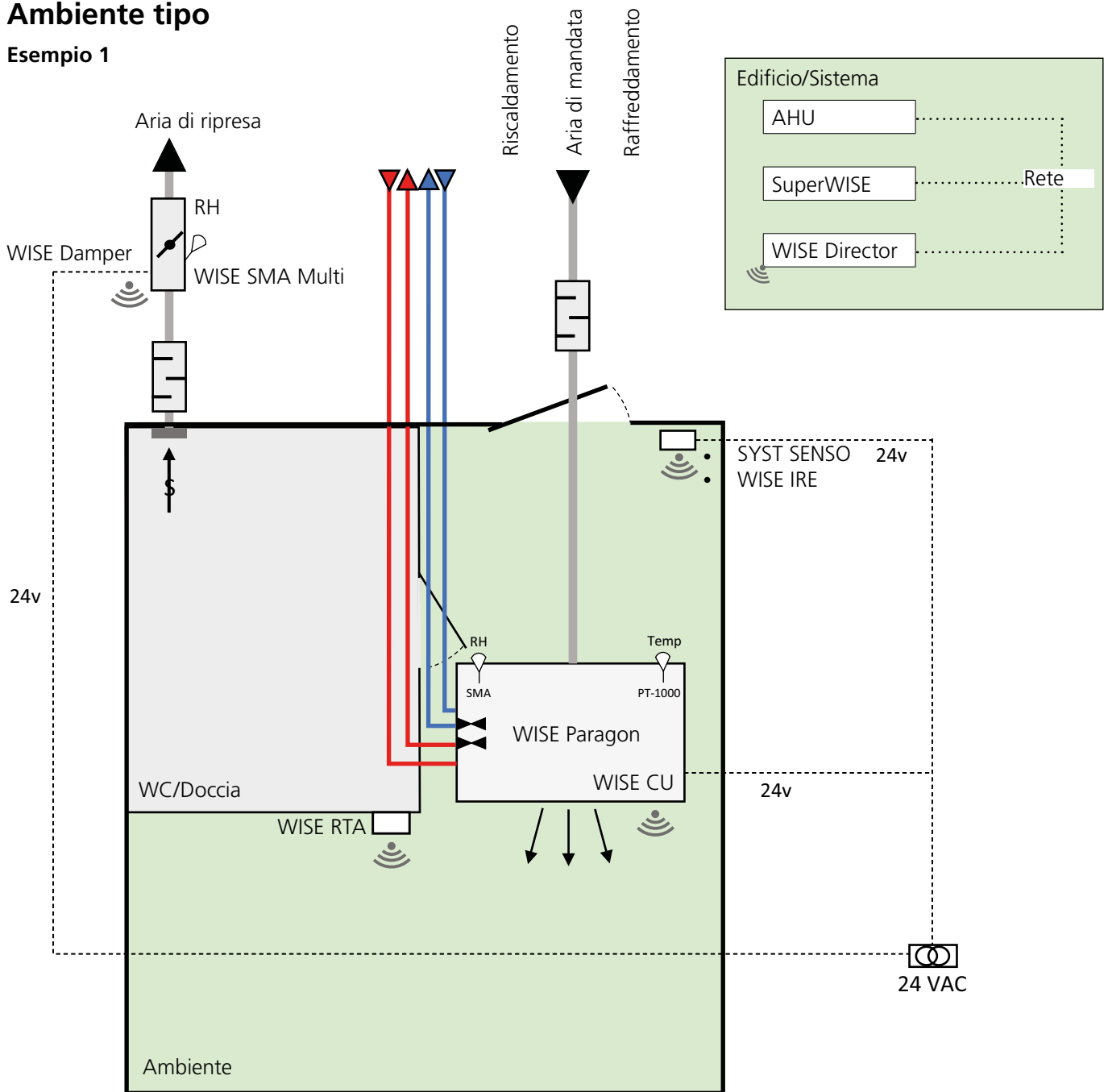
Figura 14. Soluzione per hotel con WISE Paragon, esempio 1
