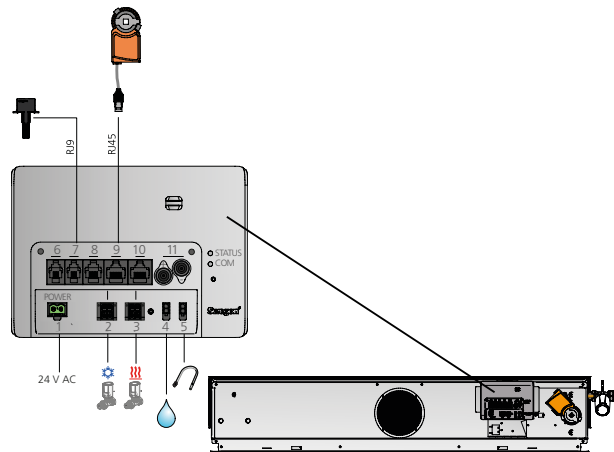
Figura 2. Componenti montati di fabbrica in WISE Paragon
