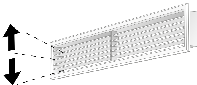
Figura 9. Distribuzione verticale dell'aria con prese d'aria regolabili nella griglia dell'aria di mandata.
