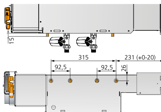
Figura 19. Dimensioni del raccordo per l'acqua
