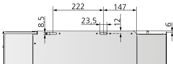
Figura 16. Dimensioni della sospensione
