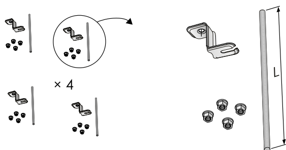
Figura 17. Raccordo di montaggio SYST MS M8-1, supporto per soffitto e asta filettata
