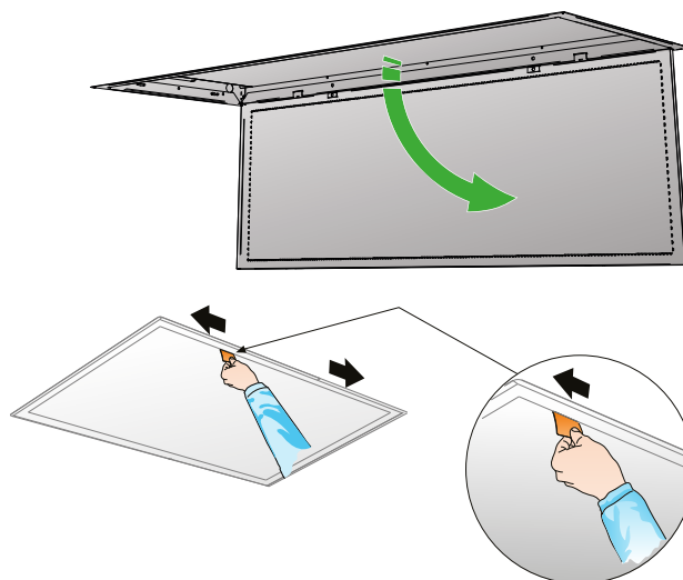
Figura 10. La griglia di ritorno è dotata di funzione di accesso rapido, che facilita la pulizia.
