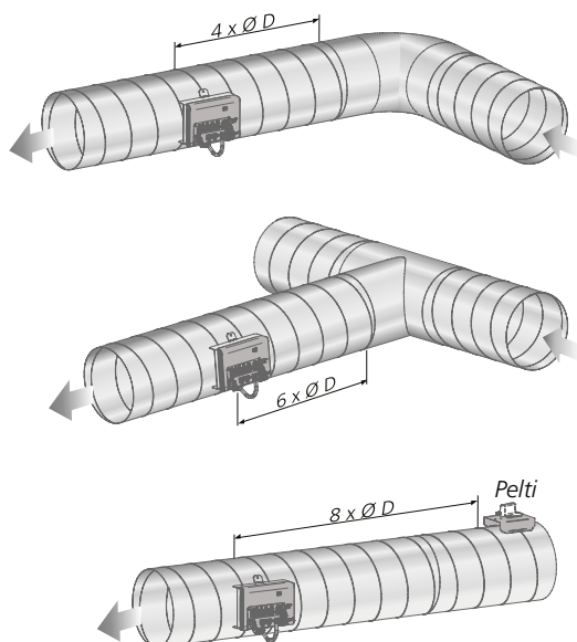
Kuva 3. Vaatimus kanavan suorasta osuudesta ennen WISE DPS.
