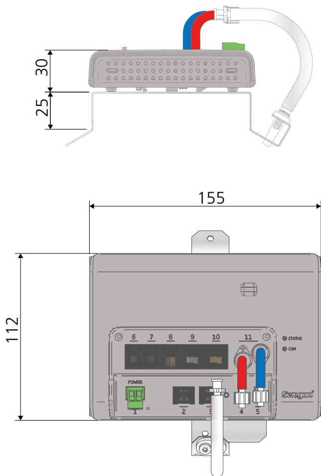
Kuva 2. Mitat, WISE DPS.
