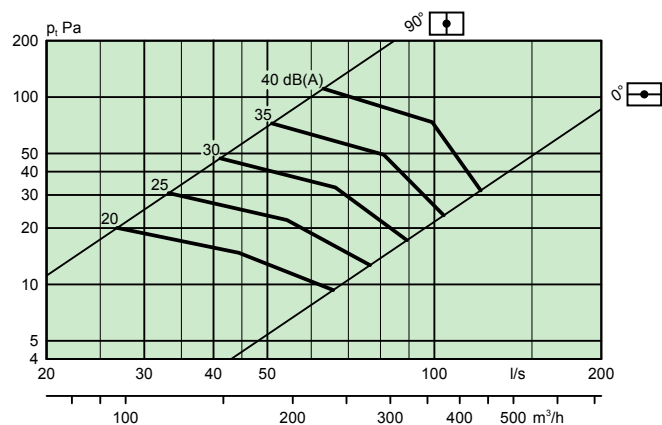
VIREO C 250 -600 + ALX 160-250 mit Klappe - Zwei Schritte
