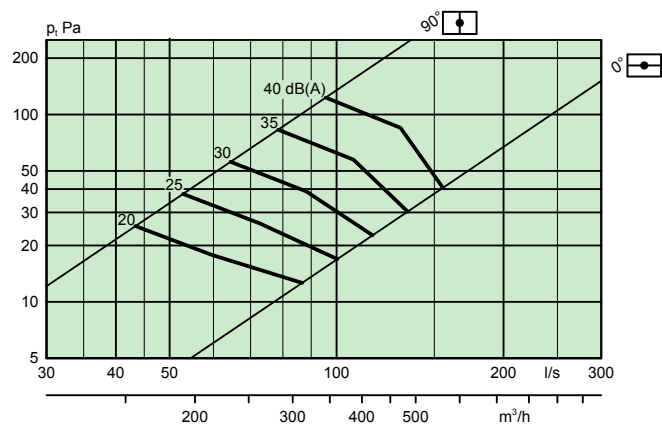
VIREO C 250 -600 + ALX 200-250 mit Klappe - Ein Schritt
