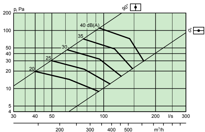
VIREO C 315 -600 + ALX 200-315 mit Klappe - Zwei Schritte
