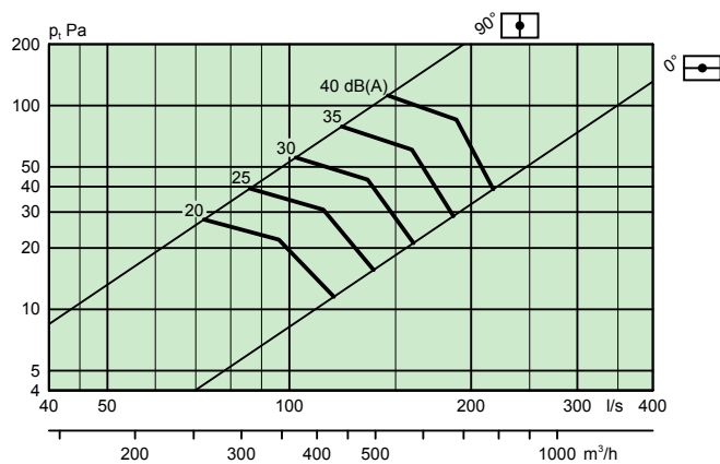
VIREO C 315 -600 + ALX 250-315 mit Klappe - Ein Schritt
