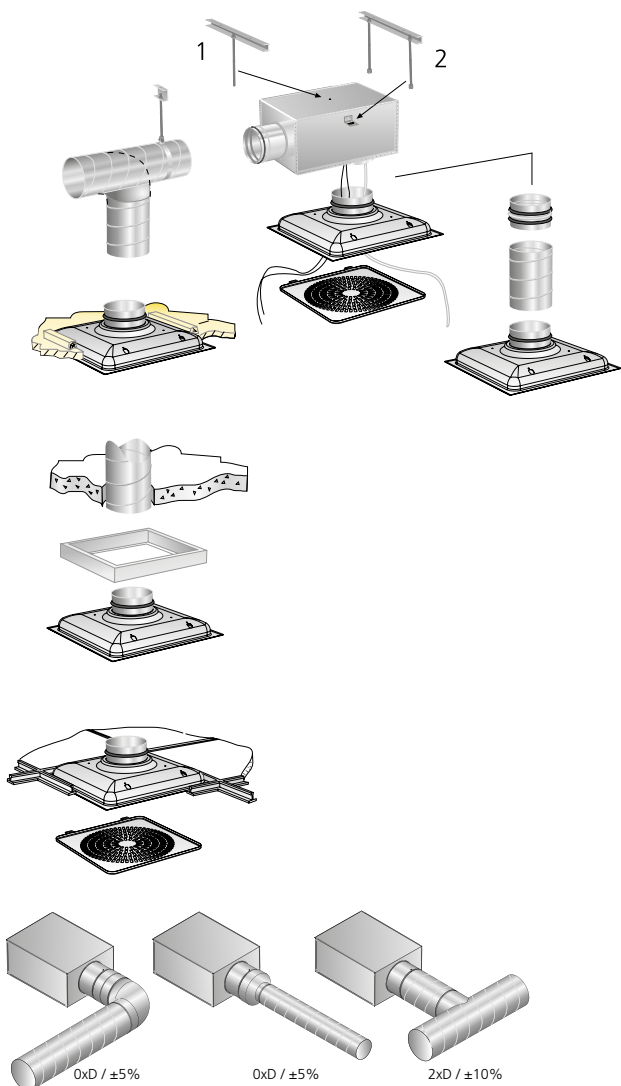
Abbildung 2. Montage.
