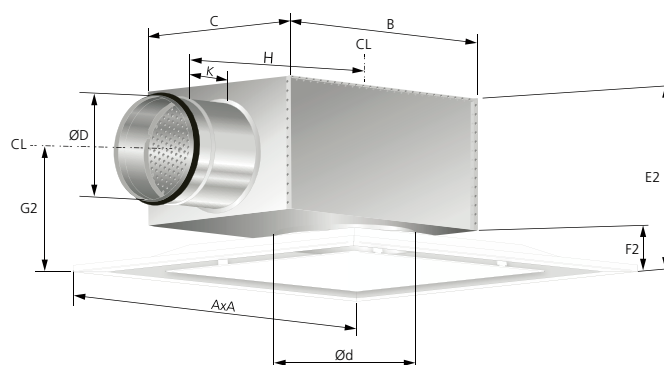
Abb. 19. KITE CR mit Anschlusskasten ALS. Niedrige Bauhöhe.
