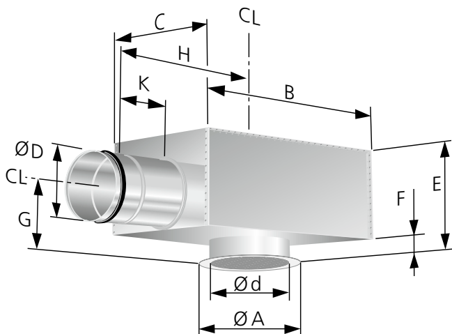
Abbildung 3. GRC mit ALS. CL = Mittellinie
