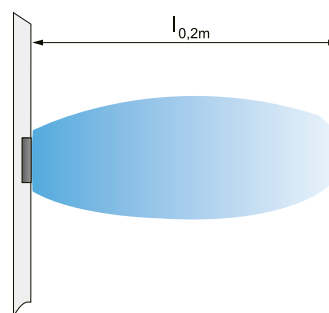
Abb. 8. Isotache. Verteilungsbild, lange Luftstromlänge (1L).
