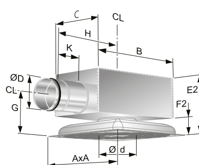
Abbildung 8. COLIBRI mit ALS. Geringe Bauhöhen.
